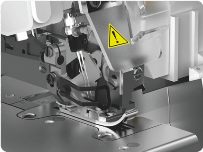
自动剪线抬压脚功能 Auto thread trimming presser foot lift
