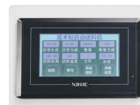
PLC控制系统，自动缝纫 PLC control system for automatic sewing
