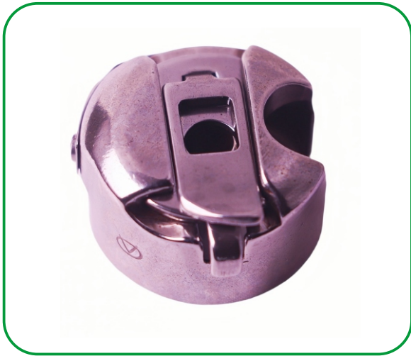
名称: 梭壳 Description: Bobbin Case 代码/Part No:10007010 适配: ZJ8700/ZJ8500/ZJ9503/ZJ9513 Machine Type: ZJ8700/ZJ8500/ZJ9503/ZJ9513
